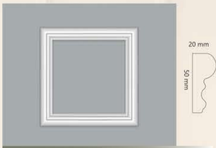
PA233-50 Profilo utilizzato JC233-W 50 x 50 cm
